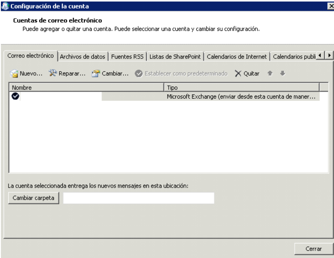
Fig.1.2; botón Nuevo...
